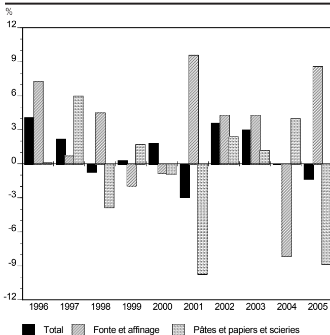
12.4A Énergie, secteur manufacturier, demande finale, selon le groupe industriel : variations
