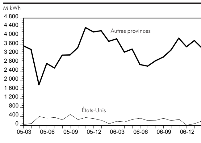
12.11A Énergie électrique, importations, selon le lieu d'origine : niveaux
